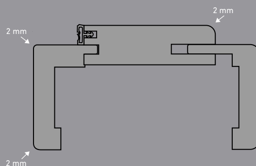
ZARGE MIT KLEINER RUNDKANTE CADRE AVEC PETIT CHANT ARRONDIS
