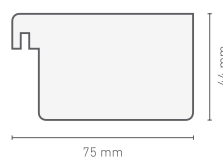
Randholz Bordure de bois
