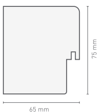
Randholz Bordure de bois
