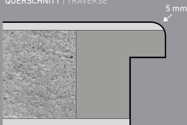
QUERSCHNITT | TRÁVERSE
