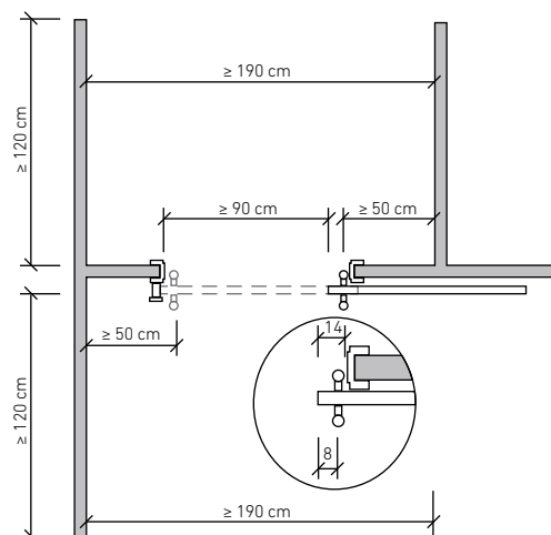
Bewegungsfläche Schiebetür
