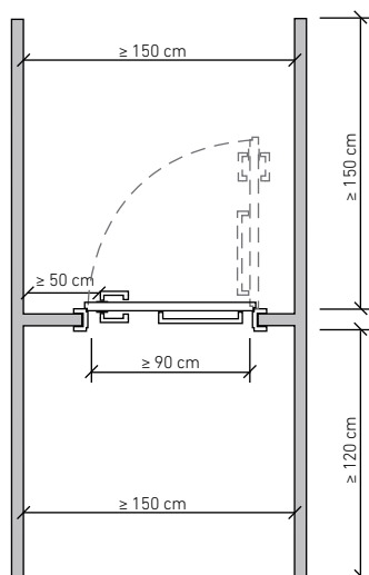
Bewegungsfläche Drehflügeltür
